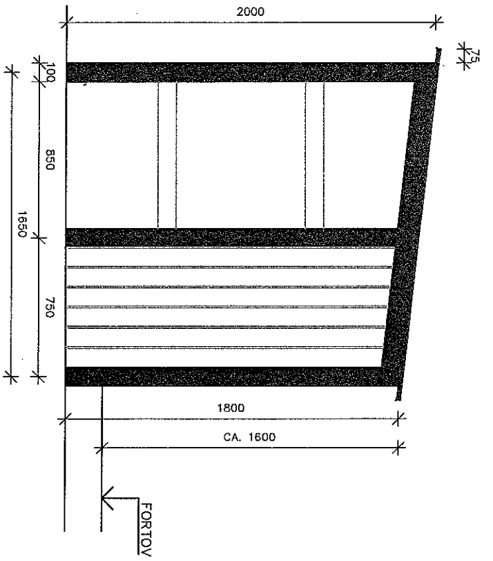
OPSTALT GAVL 1:20
