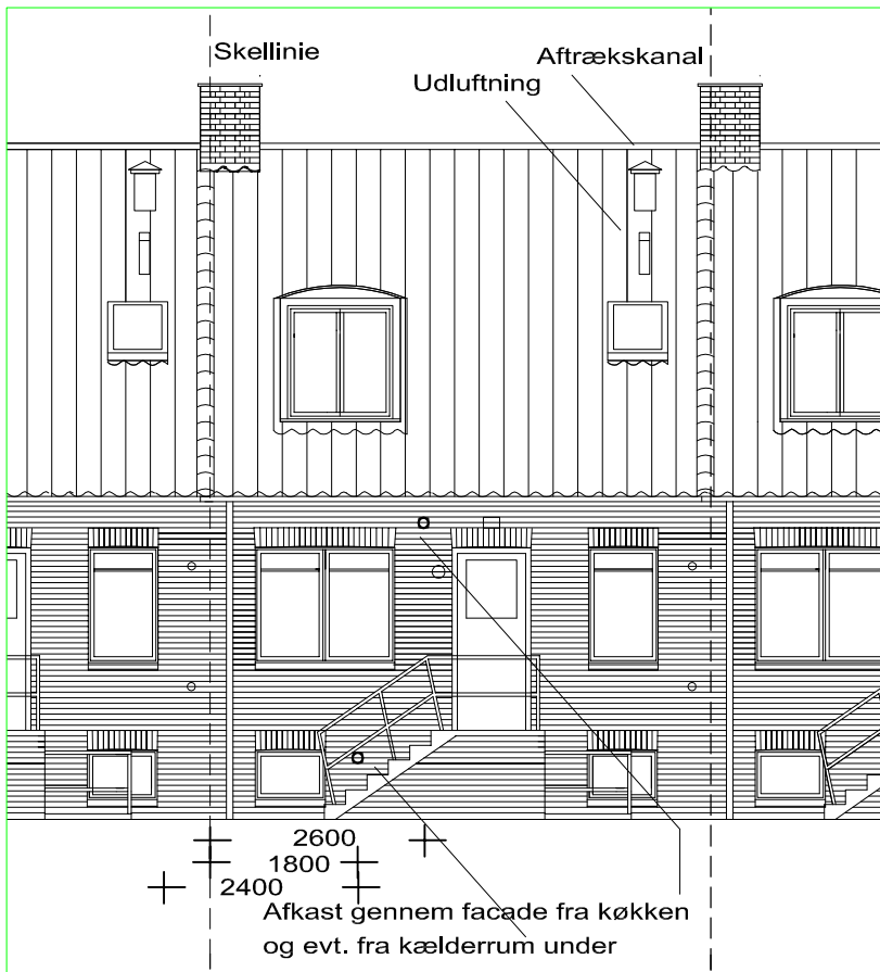
FACADE MOD GADE M. KØKKEN TV. FOR DØREN
