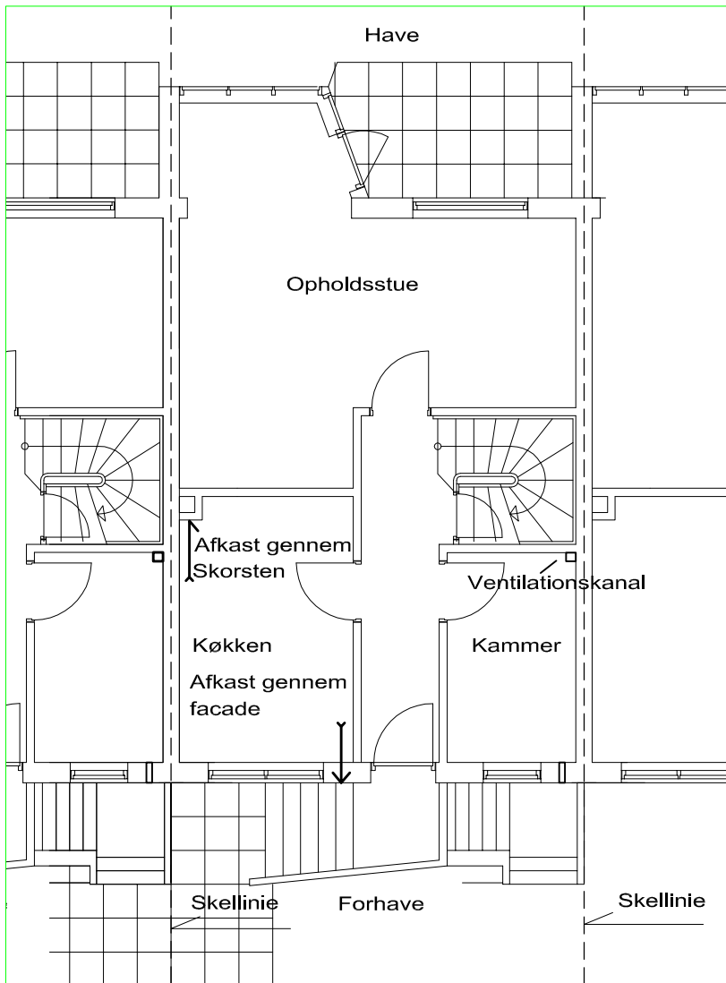
PLAN M. KØKKEN TV. FOR DØREN
