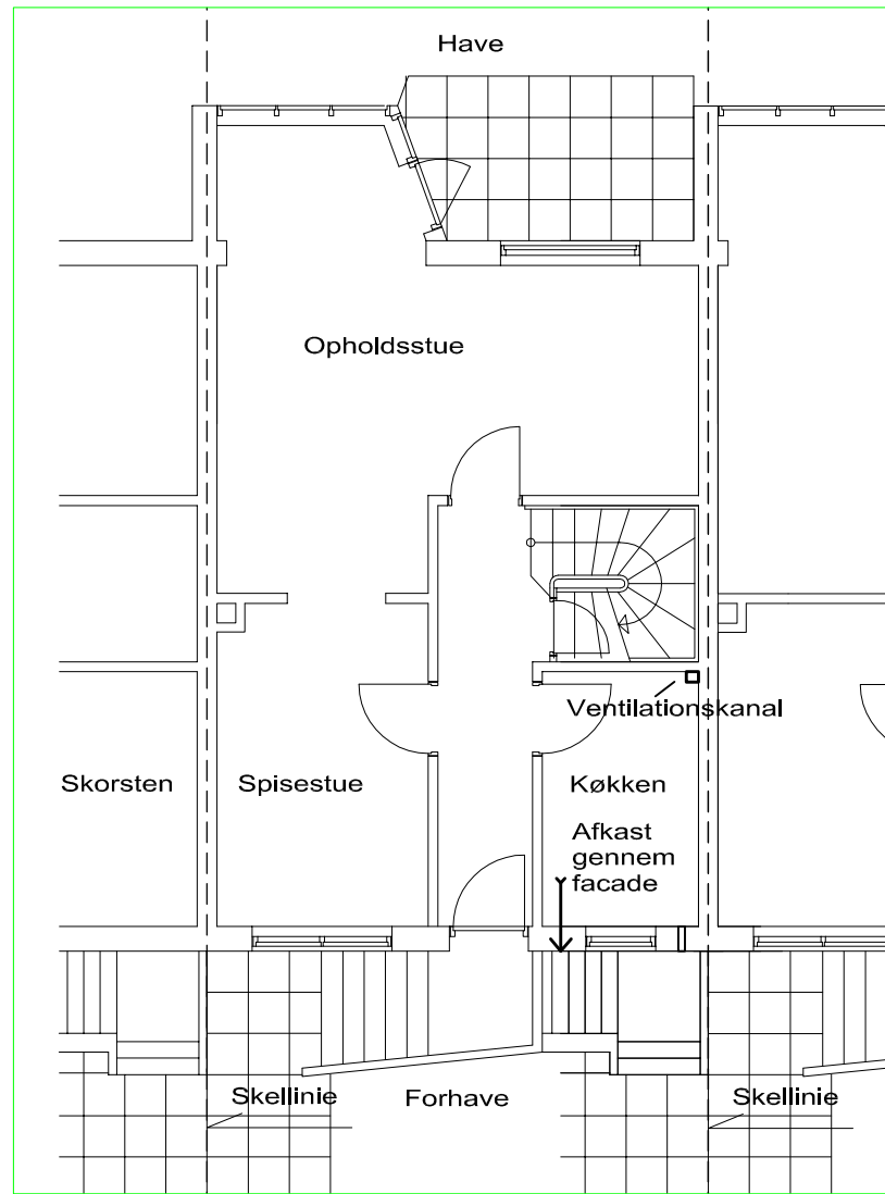
PLAN M. KØKKEN TH. FOR DØREN
