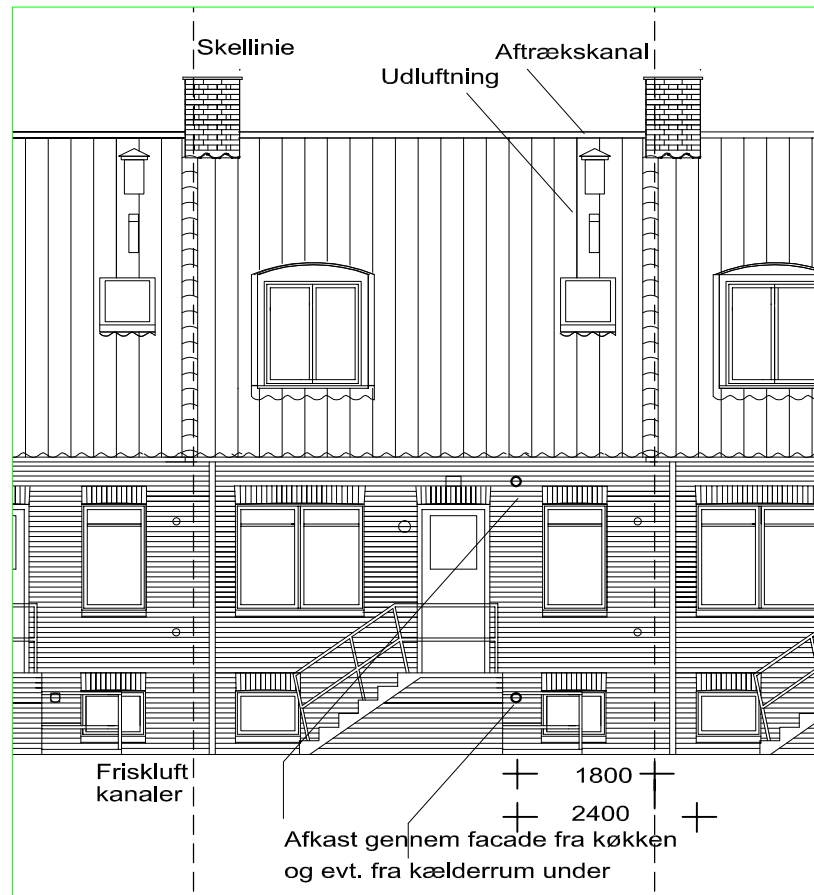
FACADE MOD GADE M. KØKKEN TH. FOR DØREN
