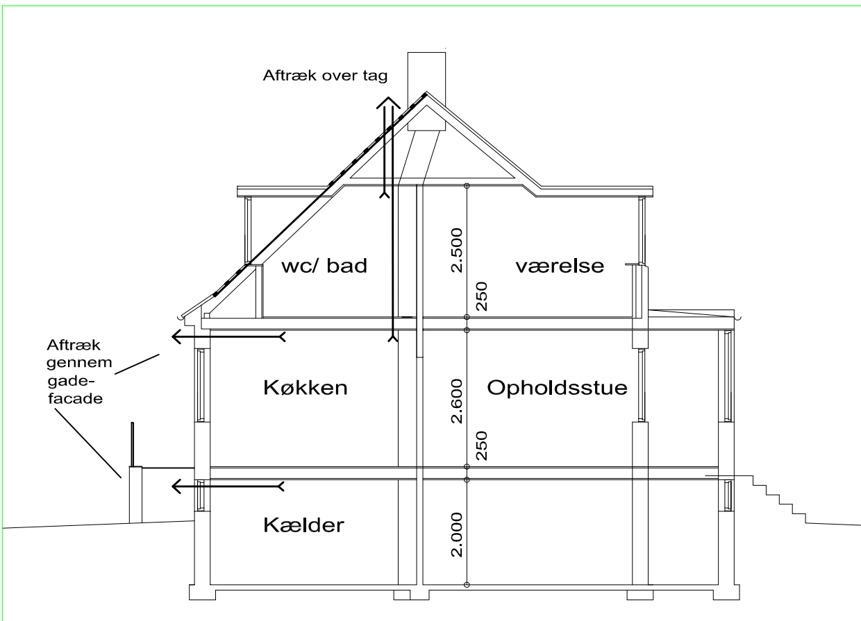
SNIT, mål 1: 100
